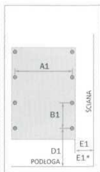
E1* Odległość panela sterującego od ściany (min.)
